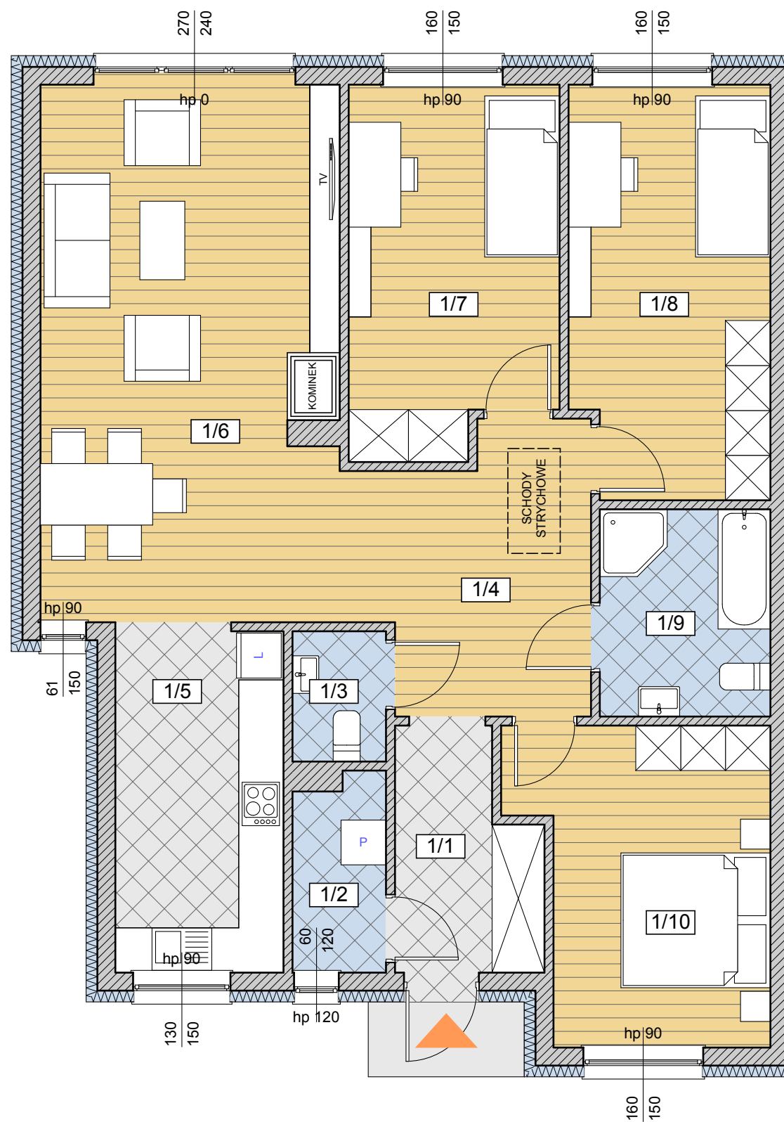
RZUT PARTERU
