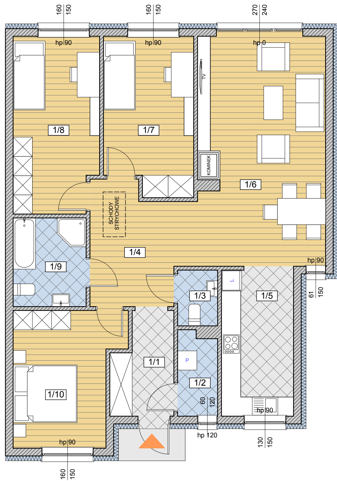
RZUT PARTERU
